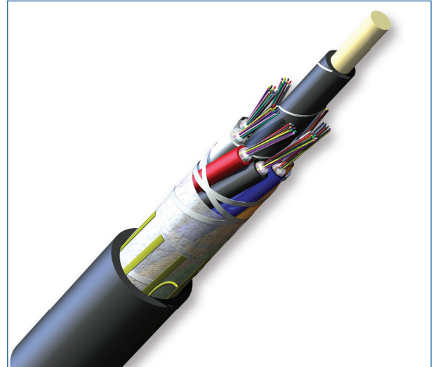
Part Number: 096KN4-T4S30A20
